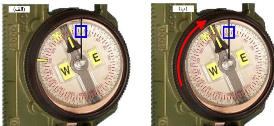
شکل ۴-۷: نحوه گرادهی به قطب‌نماهای نظامی
