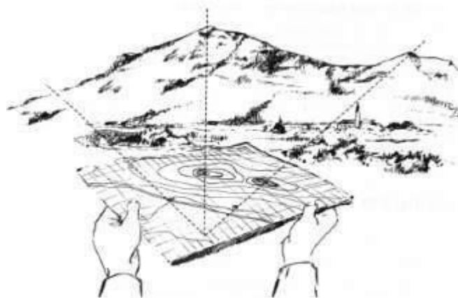
شکل ۶-۱: توجیه نقشه به روش امتدادی
